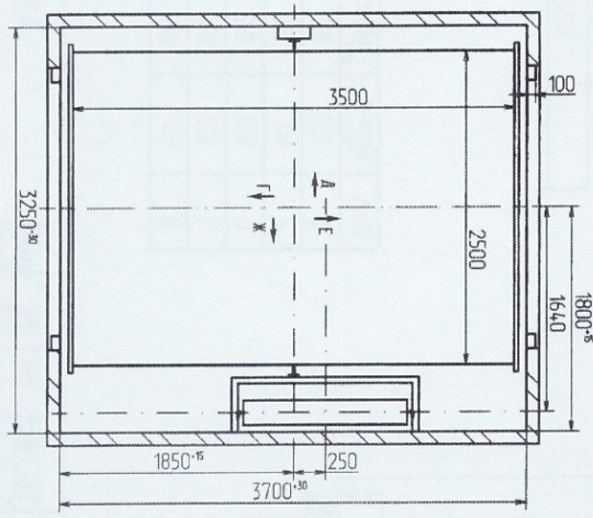
ПЛАН ШЛОЗЫ
